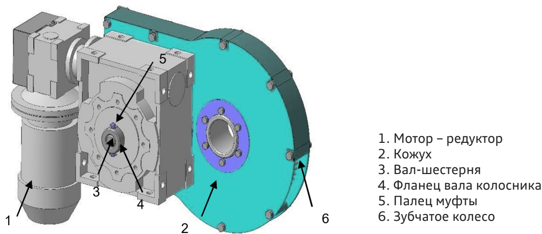
Рис.3 Привод колосника для котлов мощностью 600 – 2000 кВт
